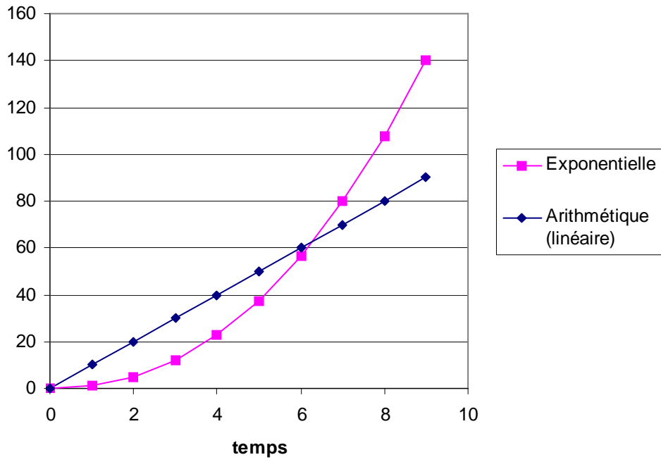
Figure 1 : croissance exponentielle vs linéaire
